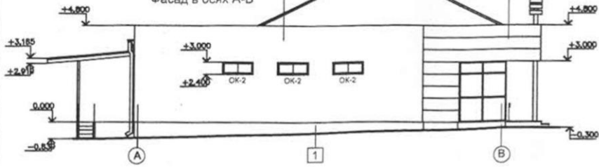
Фасад в осях А-В
